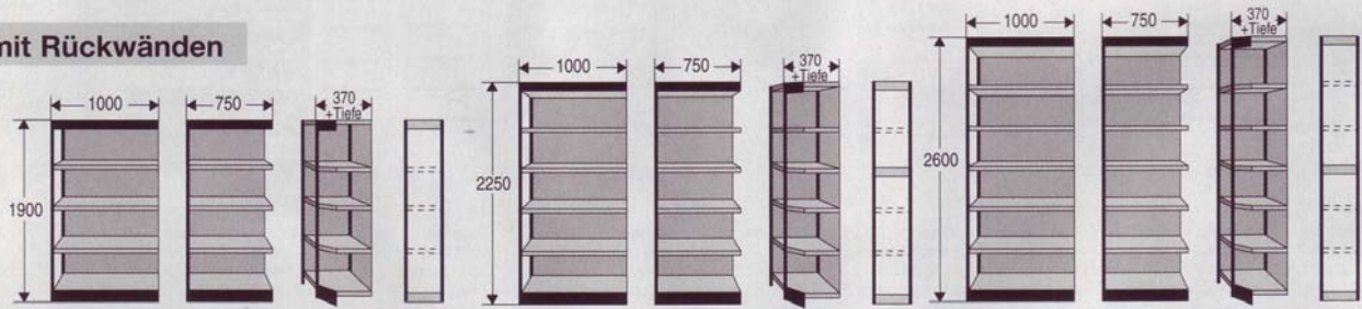
1900 mm hoch mit Rückwand und 5 Fachböden 2250 mm hoch mit Rückwand und 6 Fachböden 2600 mm hoch mit Rückwand und 7 Fachböden
