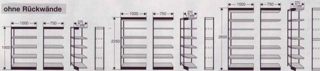
1900 mm hoch mit 5 Fachböden 2250 mm hoch mit 6 Fachböden 2600 mm hoch mit 7 Fachböden
